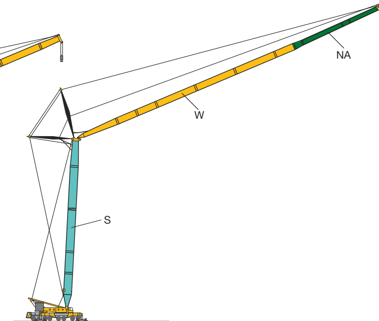
SWN 28 m – 49 m / 105 m
