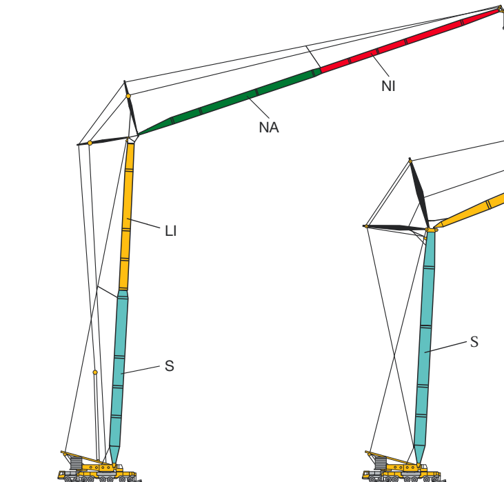
SLN 28 m – 77 m / 28 m – 91 m
